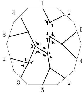
C_{12,2} : o2 - 04 - 24
