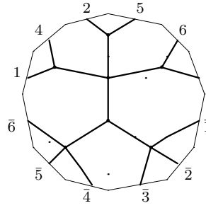
K_{4,3} : o2 - 14 - 48
