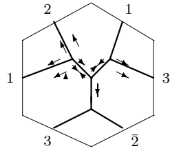
W_4 : q2 - 02 - 12
