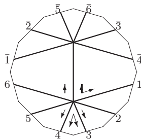
L_7 : o3 - 04 - 07
