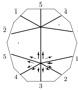
L_6 : o1 - 02 - 12
