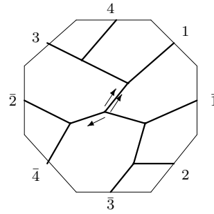
C_{9,1} : o1 - 05 - 18
