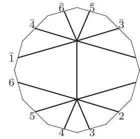
L_7 : o2 - 18 - 28
