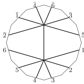
L_7 : o2 - 22 - 28
