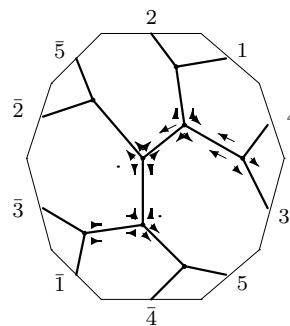
C_{12,3} : o2 - 12 - 24
