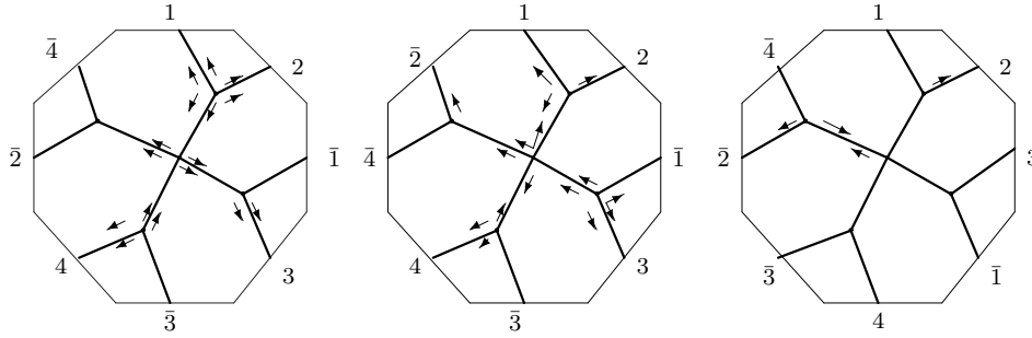
W_5 : o1 - 01 - 16
