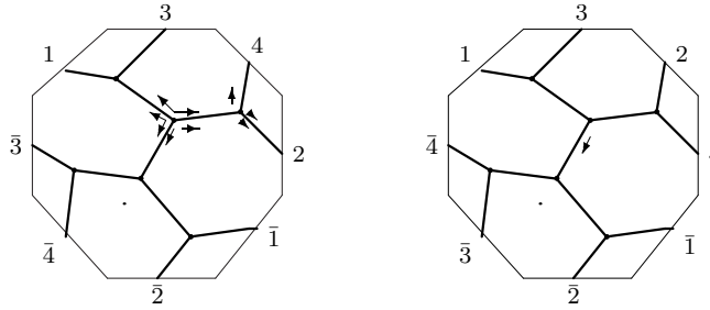
K_{3,3} : o1 - 01 - 09
