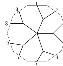
W_6 : o1 - 11 - 40
