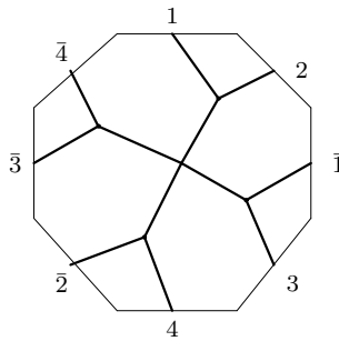
W_5 : o2 - 02 - 08
