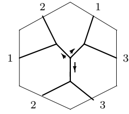
W_4 : q2 - 03 - 03
