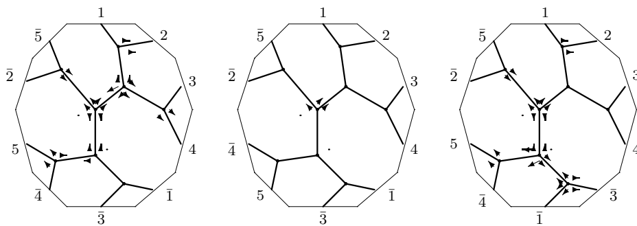
C_{12,3} : o2 - 01 - 24
