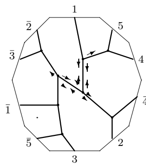
C_{12,4} : o1 - 02 - 12
