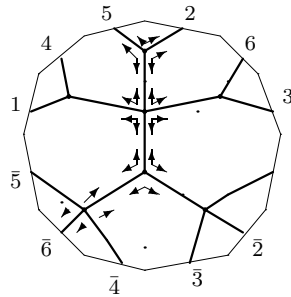
K_{4,3} : o3 - 02 - 24
