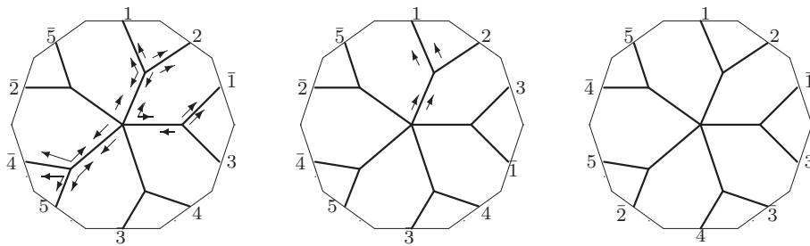
W_6 : o2 - 04 - 20
