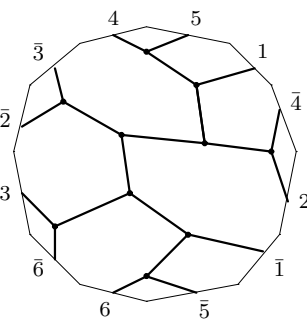
C_{15,11} : o2 - 03 - 60
