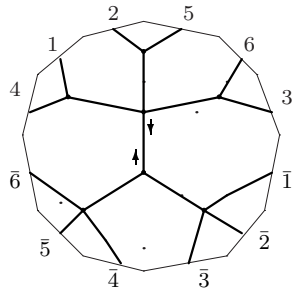
K_{4,3} : o2 - 01 - 02
