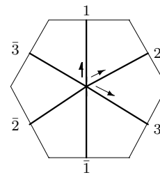
B_3 : o1 - 03 - 03
