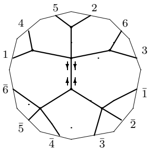
K_{4,3} : o2 - 09 - 04
