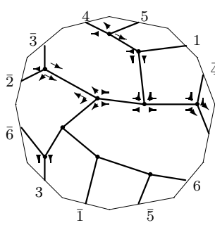
C_{15,11} : o2 - 20 - 30
