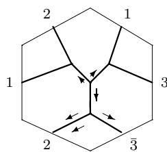
W_4 : q1 - 01 - 06
