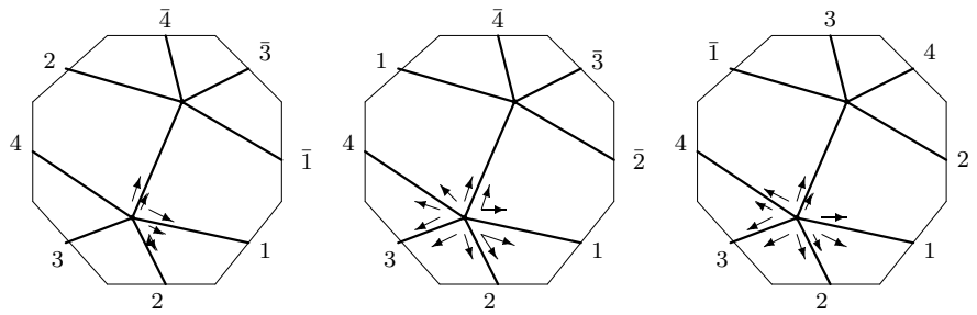
L_5 : q2 - 01 - 05
