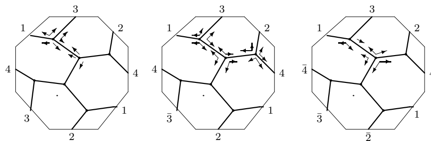
K_{3,3} : q3 - 04 - 09
