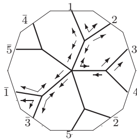
W_6 : o2 - 37 - 20
