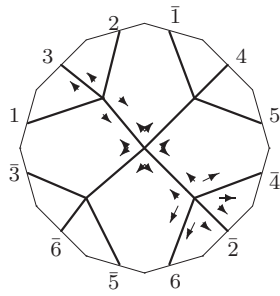
K_5 : o2 - 28 - 20
