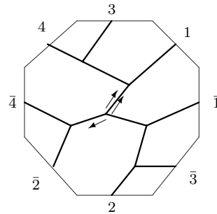
C_{9,1} : o0 - 01 - 03
