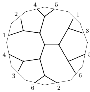
C_{15,14} : o3 - 01 - 60
