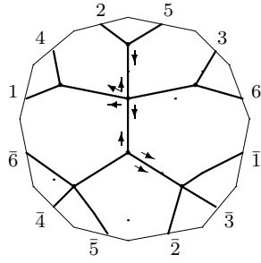
K_{4,3} : o2 - 15 - 08
