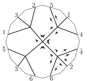
W_6 : o1 - 05 - 20
