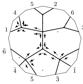
K_{4,3} : o2 - 04 - 24
