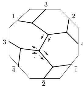
K_{3,3} : o2 - 01 - 06
