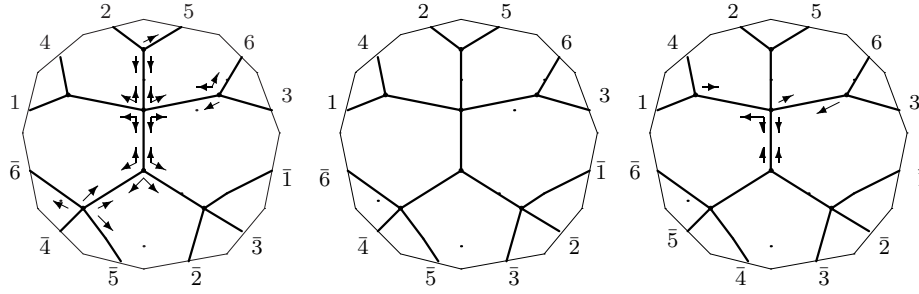
K_{4,3} : o3 - 04 - 24
