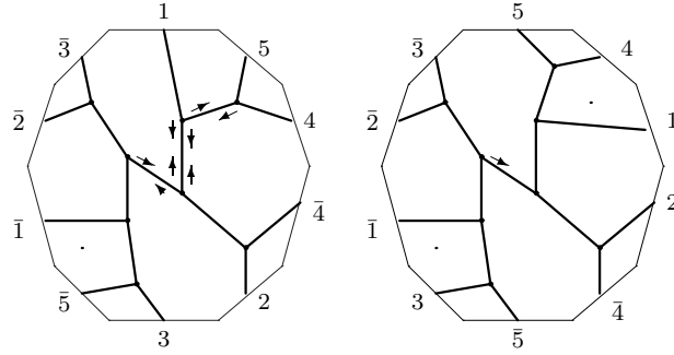
C_{12,4} : o1 - 04 - 08
