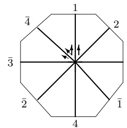
B_4 : o1 - 06 - 08
