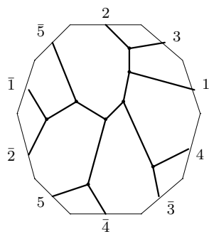
C_{12,1} : o2 - 05 - 48
