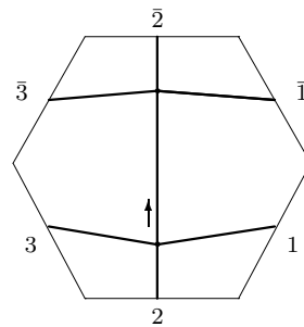
L_4 : o0 - 01 - 01
