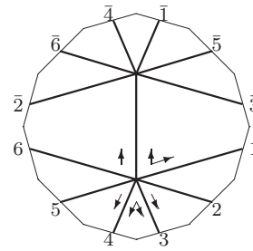
L_7 : o3 - 15 - 07
