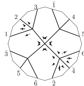
K_5 : o2 - 12 - 20
