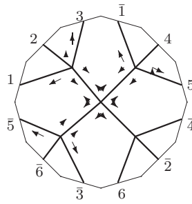
K_5 : o3 - 05 - 20
