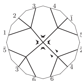
K_5 : o1 - 03 - 10
