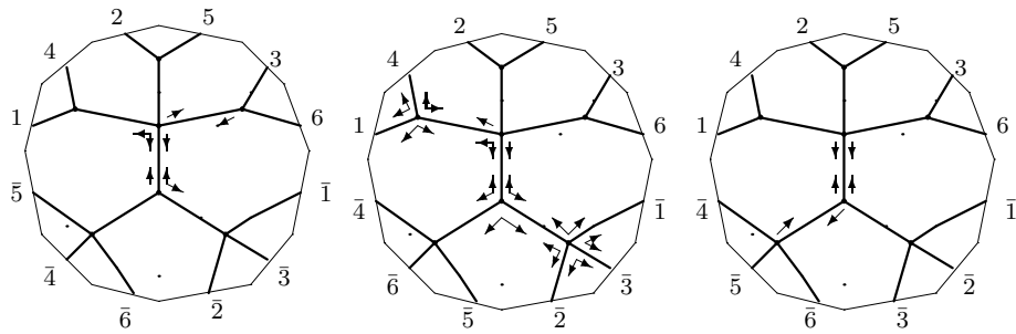
K_{4,3} : o3 - 07 - 08
