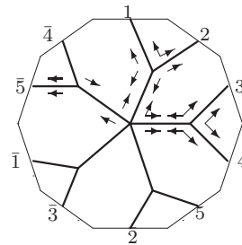
W_6 : o2 - 39 - 20
