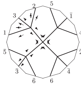
K_5 : o2 - 31 - 20
