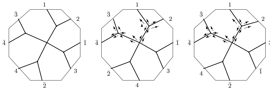
W_5 : o1 - 04 - 32
