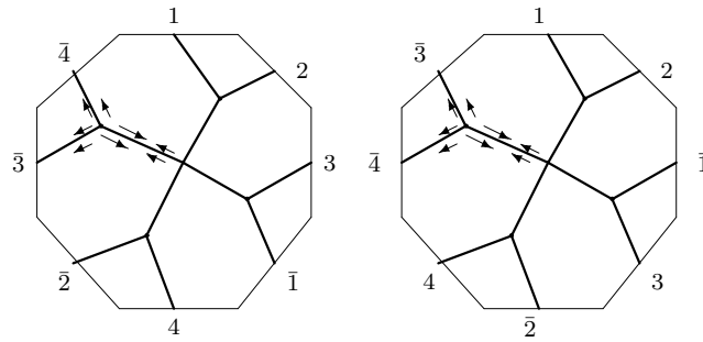
W_5 : o1 - 04 - 32
