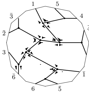
C_{15,11} : o2 - 11 - 30
