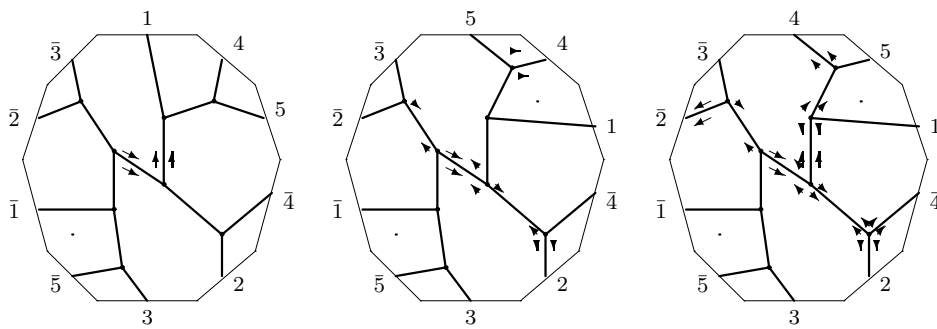
C_{12,4} : o2 - 04 - 04
