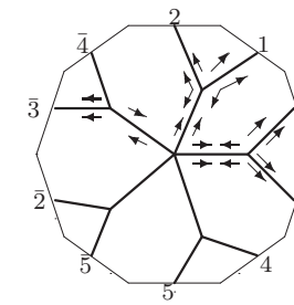
W_6 : o1 - 12 - 20
