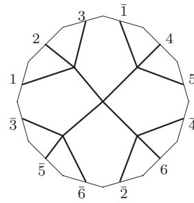
K_5 : o3 - 06 - 40
