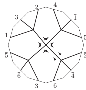
K_5 : o2 - 30 - 10
