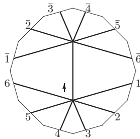
L_7 : o3 - 01 - 01
