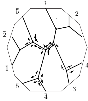
C_{12,1} : o2 - 07 - 24
