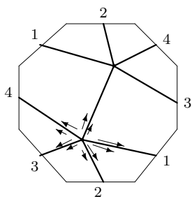
L_5 : q3 - 05 - 20
