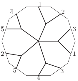
W_6 : o2 - 14 - 40
