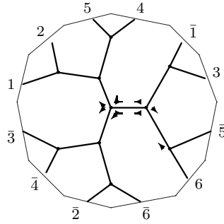
C_{15,14} : o1 - 01 - 10
