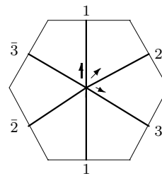
B_3 : q3 - 08 - 03
