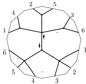
K_{4,3} : o3 - 10 - 02
