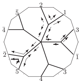
W_6 : o2 - 19 - 20
