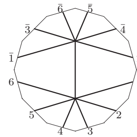
L_7 : o2 - 15 - 28
