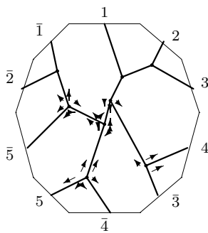
C_{12,1} : o1 - 11 - 24
