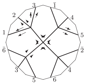
K_5 : o2 - 02 - 20
