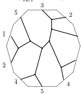
C_{12,1} : o2 - 13 - 24
