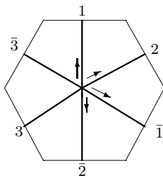
B_3 : o1 - 01 - 04
