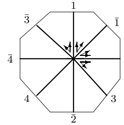
B_4 : o1 - 03 - 08
