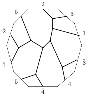
C_{12,1} : o2 - 01 - 28
