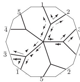
W_6 : o2 - 35 - 20
