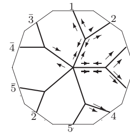
W_6 : o1 - 09 - 20
