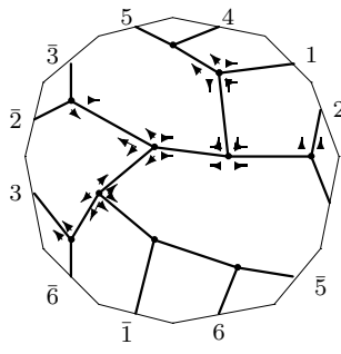
C_{15,11} : o2 - 25 - 30
