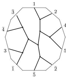
C_{12,2} : o2 - 02 - 48
