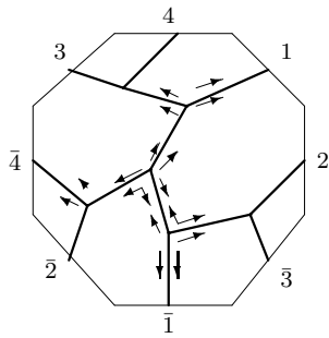
C_{9,1} : o2 - 01 - 18
