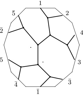
C_{12,3} : o2 - 05 - 48
