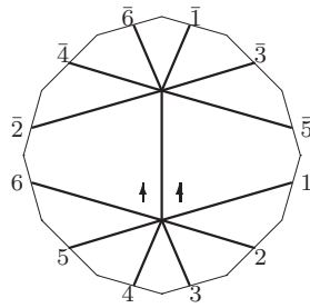
L_7 : o3 - 13 - 02
