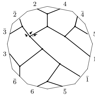
C_{15,11} : o0 - 01 - 03
