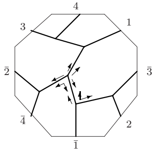
C_{9,1} : o1 - 04 - 09
