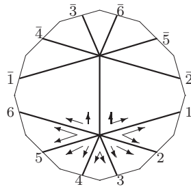
L_7 : o2 - 16 - 14
