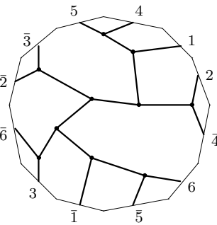
C_{15,11} : o3 - 02 - 60
