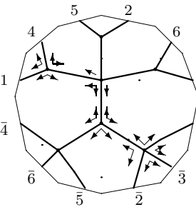
K_{4,3} : o2 - 05 - 24
