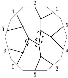
C_{12,2} : o1 - 01 - 08
