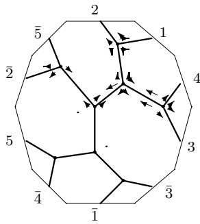
C_{12,3} : o2 - 08 - 24
