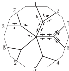
W_6 : o2 - 20 - 20
