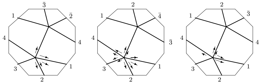
L_5 : q2 - 01 - 05
