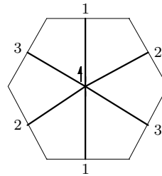
B_3 : q1 - 05 - 01
