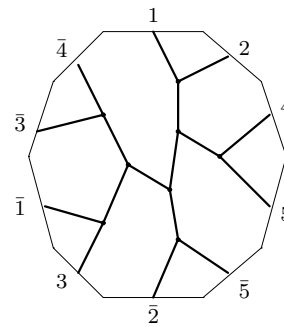
C_{12,2} : o2 - 09 - 48
