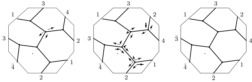
K_{3,3} : q4 - 01 - 03
