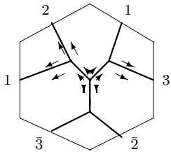
W_4 : q3 - 01 - 12
