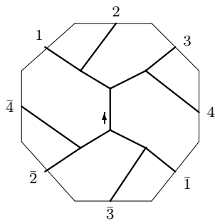
C_{9,2} : o1 - 01 - 01
