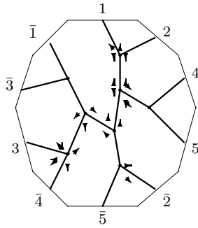
C_{12,2} : o1 - 02 - 24
