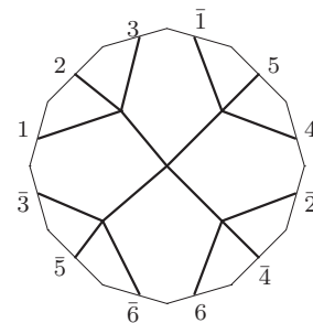
K_5 : o2 - 15 - 40
