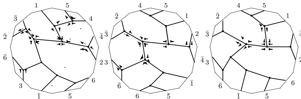
C_{15,11} : o1 - 01 - 30
