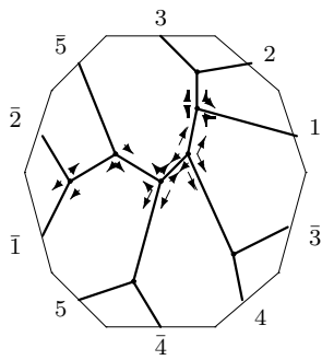
C_{12,1} : o1 - 01 - 24
