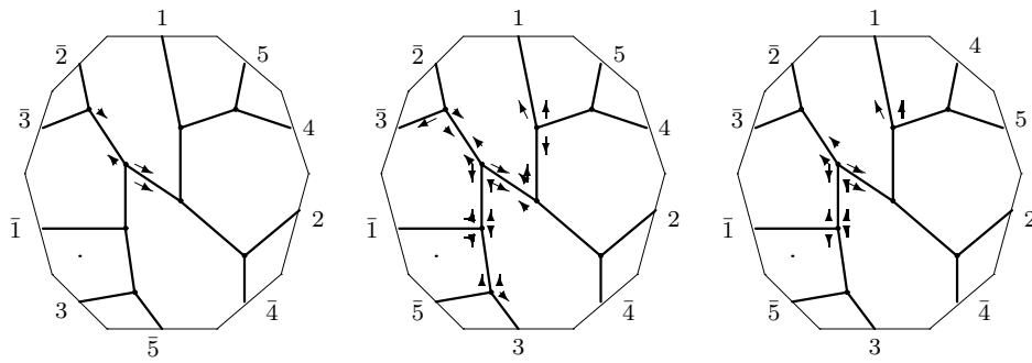
C_{12,4} : o2 - 01 - 04
