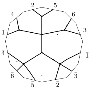
K_{4,3} : o2 - 12 - 48
