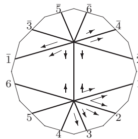
L_7 : o3 - 06 - 14
