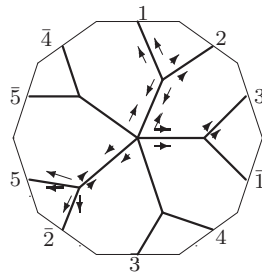
W_6 : o1 - 05 - 20
