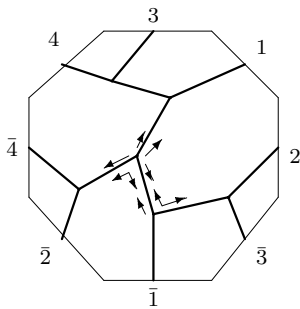
C_{9,1} : o1 - 01 - 09
