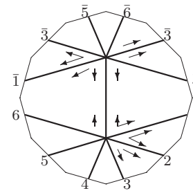
L_7 : o2 - 12 - 14
