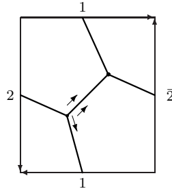
L_3 : q2 - 01 - 03
