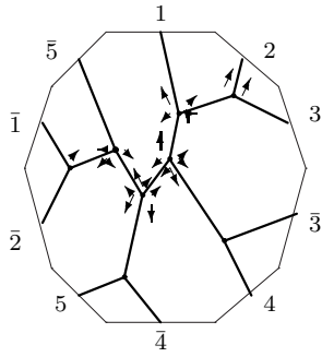
C_{12,1} : o1 - 04 - 24
