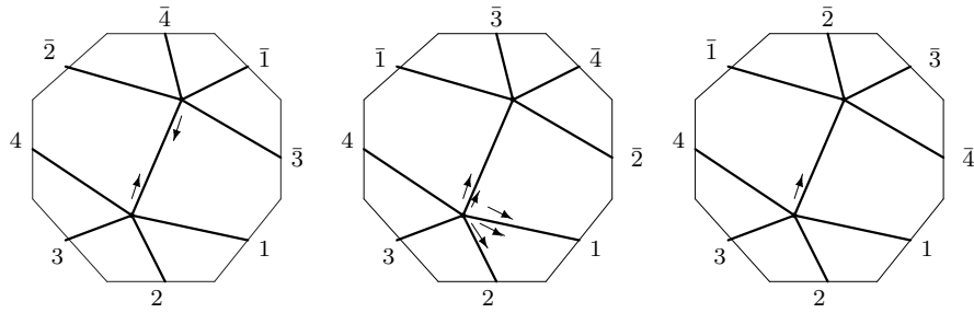
L_5 : o2 - 01 - 02
