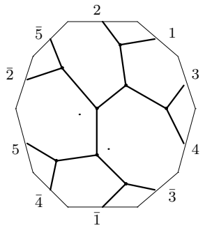
C_{12,3} : o2 - 07 - 48
