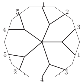
W_6 : o2 - 11 - 40
