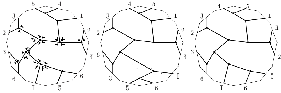
C_{15,11} : o3 - 04 - 30
