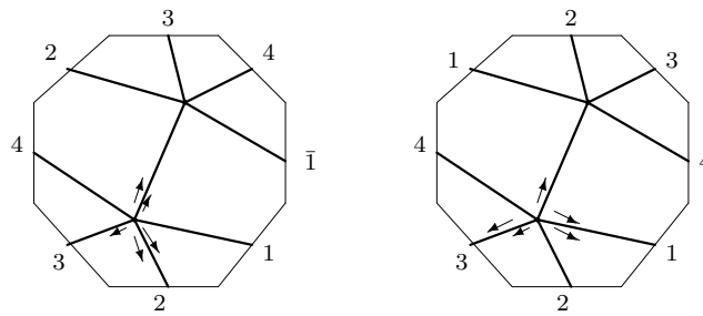
L_5 : q1 - 01 - 05
