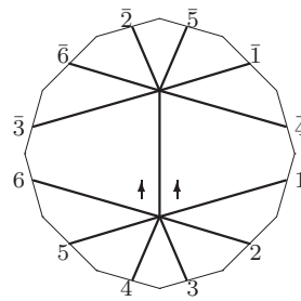
L_7 : o3 - 16 - 02
