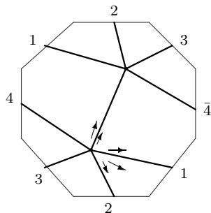
L_5 : q2 - 07 - 05
