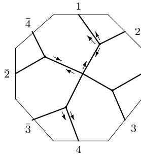
W_5 : o2 - 02 - 08
