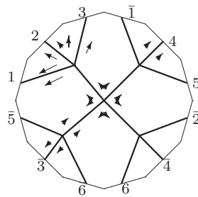
K_5 : o2 - 03 - 20
