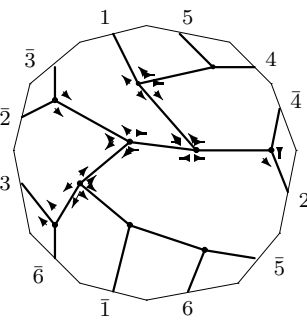
C_{15,11} : o2 - 09 - 30
