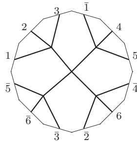
K_5 : o2 - 08 - 40
