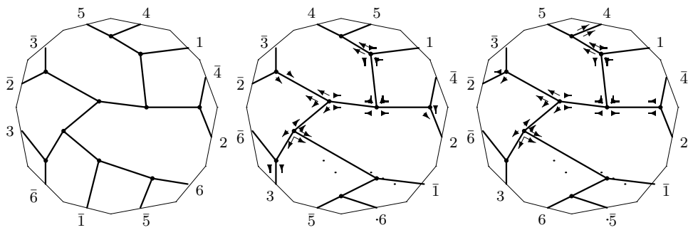
C_{15,11} : o3 - 07 - 60
