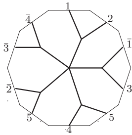
W_6 : o2 - 31 - 40
