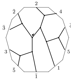
C_{12,4} : o0 - 01 - 01
