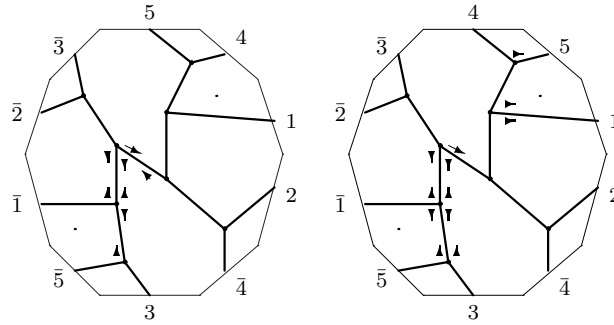
C_{12,4} : o2 - 07 - 08
