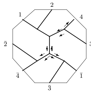
C_{9,2} : o1 - 02 - 09
