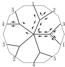
W_6 : o2 - 28 - 20
