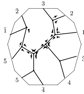
C_{12,1} : o1 - 06 - 24
