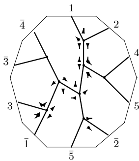
C_{12,2} : o2 - 01 - 24
