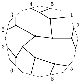
C_{15,11} : o3 - 03 - 60
