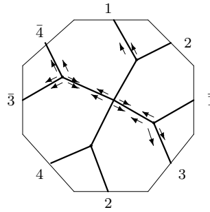
W_5 : o2 - 03 - 16
