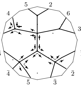
K_{4,3} : o2 - 08 - 24
