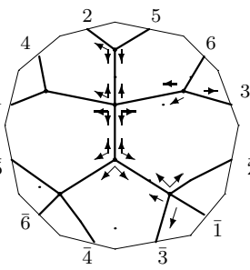
K_{4,3} : o2 - 11 - 24
