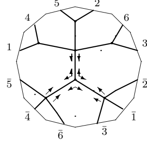
K_{4,3} : o2 - 03 - 12
