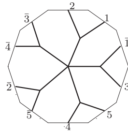
W_6 : o2 - 32 - 40
