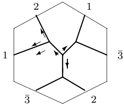
W_4 : q2 - 01 - 06
