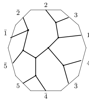
C_{12,1} : o1 - 09 - 48
