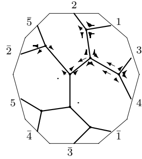
C_{12,3} : o2 - 06 - 24
