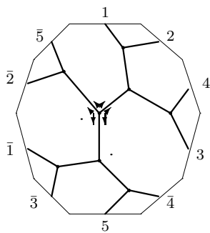
C_{12,3} : o2 - 10 - 06
