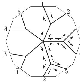
W_6 : o2 - 38 - 20
