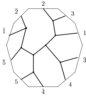
C_{12,1} : o1 - 05 - 48
