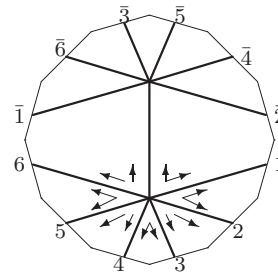
L_7 : o2 - 20 - 14
