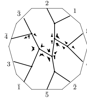
C_{12,2} : o2 - 06 - 24
