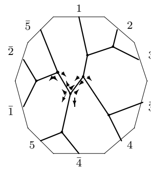
C_{12,1} : o1 - 03 - 12
