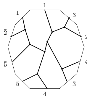
C_{12,1} : o1 - 12 - 48
