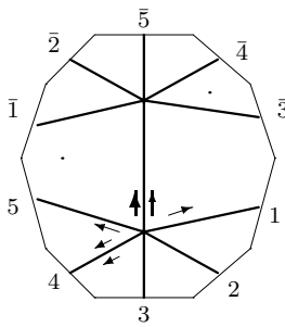
L_6 : o1 - 06 - 06
