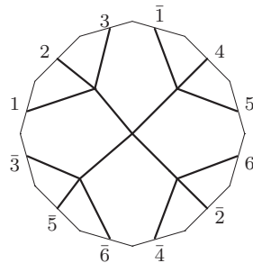
K_5 : o2 - 11 - 40
