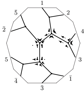
C_{12,3} : o2 - 04 - 24
