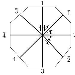
B_4 : o0 - 02 - 08
