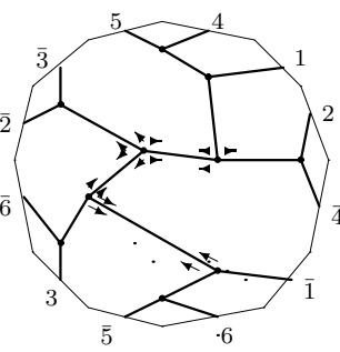
C_{15,11} : o2 - 23 - 15
