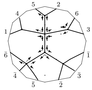
K_{4,3} : o2 - 06 - 24
