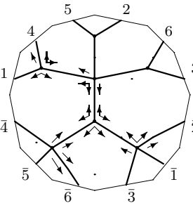
K_{4,3} : o2 - 02 - 24
