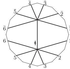
L_7 : o0 - 01 - 01
