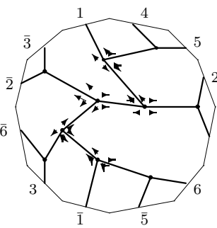
C_{15,11} : o2 - 06 - 30
