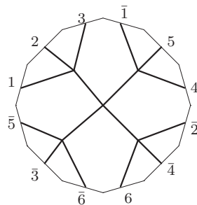
K_5 : o2 - 14 - 40
