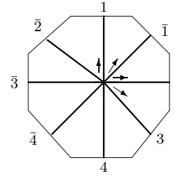
B_4 : o0 - 03 - 04
