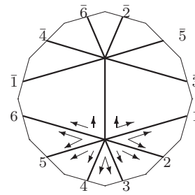
L_7 : o3 - 09 - 14
