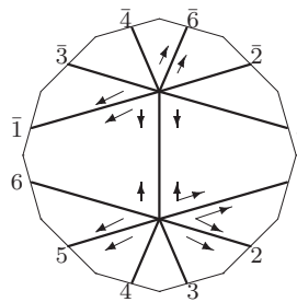
L_7 : o3 - 05 - 14
