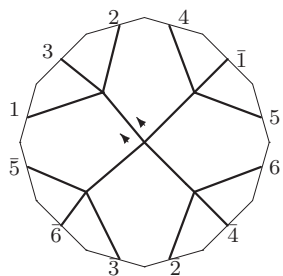
K_5 : o1 - 04 - 02
