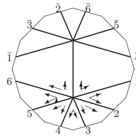
L_7 : o1 - 02 - 14
