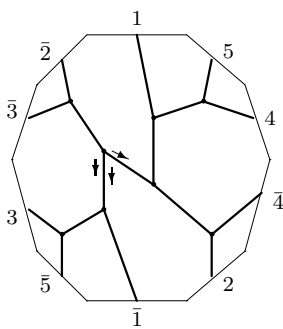
C_{12,4} : o1 - 01 - 03
