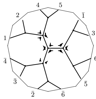
C_{15,14} : o3 - 02 - 20
