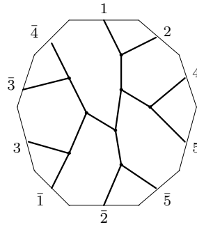
C_{12,2} : o1 - 03 - 48
