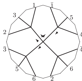
W_6 : o1 - 06 - 05
