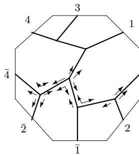
C_{9,1} : o1 - 02 - 18
