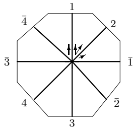
B_4 : o2 - 01 - 04
