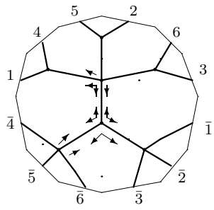
K_{4,3} : o2 - 07 - 12
