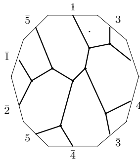
C_{12,1} : o2 - 07 - 24
