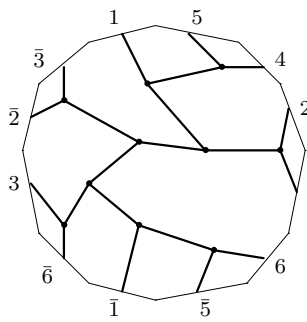
C_{15,11} : o2 - 07 - 60
