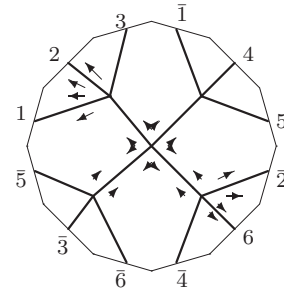
K_5 : o2 - 06 - 20
