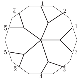
W_6 : o1 - 03 - 40
