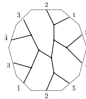
C_{12,2} : o2 - 12 - 48
