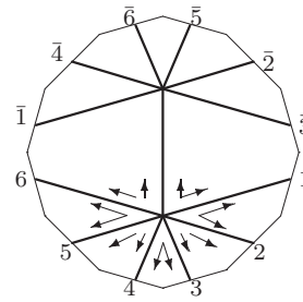
L_7 : o2 - 17 - 14
