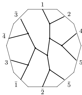
C_{12,2} : o1 - 04 - 48
