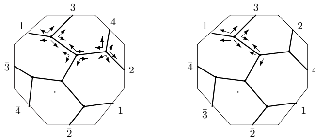
K_{3,3} : q2 - 01 - 18
