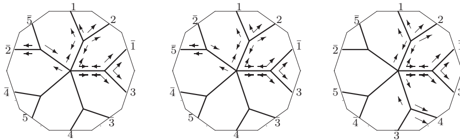
W_6 : o2 - 01 - 20
