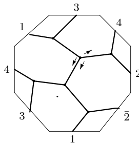
K_{3,3} : q1 - 01 - 03
