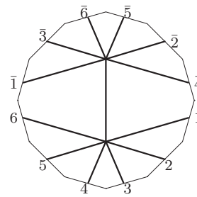
L_7 : o2 - 14 - 28
