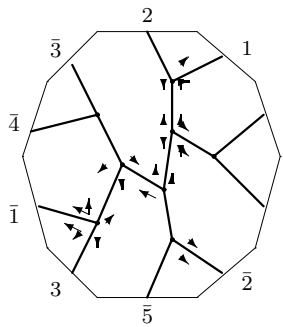
C_{12,2} : o2 - 07 - 24
