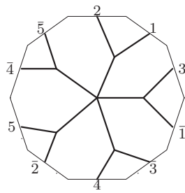
W_6 : o2 - 17 - 40
