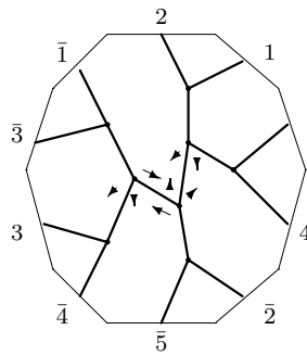
C_{12,2} : o2 - 08 - 08
