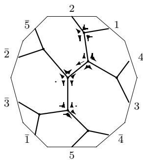
C_{12,3} : o2 - 11 - 24
