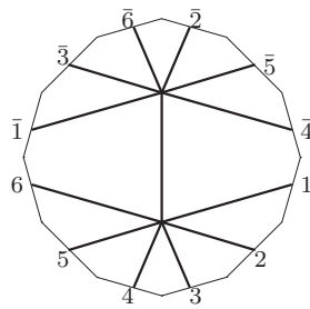
L_7 : o2 - 13 - 28
