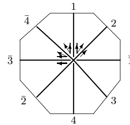
B_4 : o2 - 03 - 08
