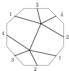
L_5 : q3 - 02 - 20
