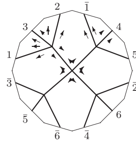
K_5 : o3 - 12 - 20
