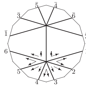
L_7 : o2 - 11 - 14
