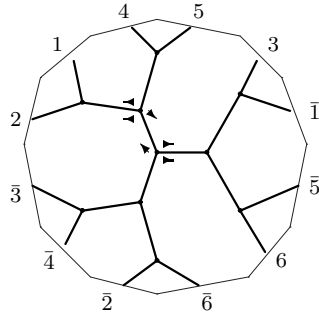
C_{15,14} : o2 - 07 - 06
