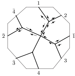
W_5 : o2 - 01 - 16
