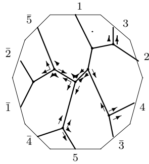
C_{12,1} : o2 - 21 - 24
