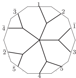
W_6 : o2 - 25 - 40
