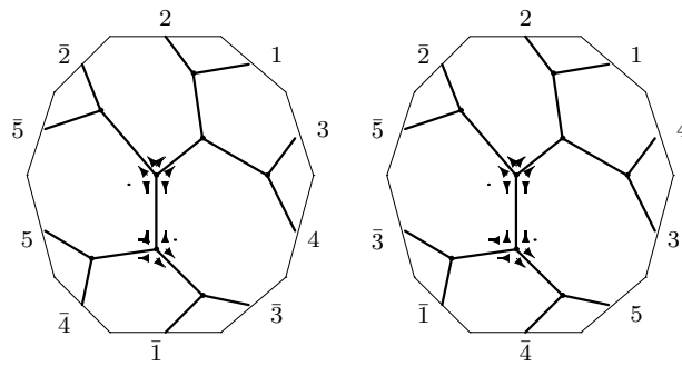
C_{12,3} : o1 - 04 - 12
