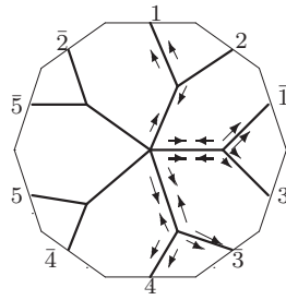
W_6 : o1 - 02 - 20
