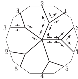
W_6 : o2 - 33 - 20
