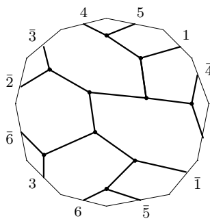
C_{15,11} : o2 - 01 - 60
