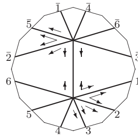
L_7 : o3 - 14 - 14
