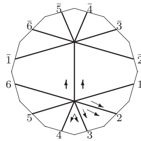
L_7 : o1 - 03 - 07
