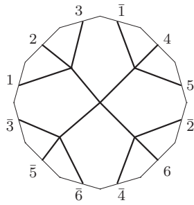
K_5 : o3 - 04 - 40
