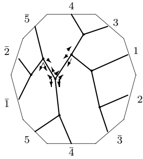
C_{12,1} : o1 - 13 - 12
