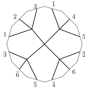
K_5 : o2 - 05 - 40
