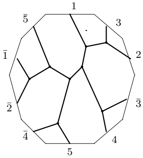
C_{12,1} : o2 - 20 - 48
