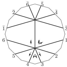
L_7 : o1 - 01 - 07
