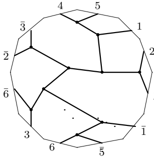
C_{15,11} : o2 - 24 - 60
