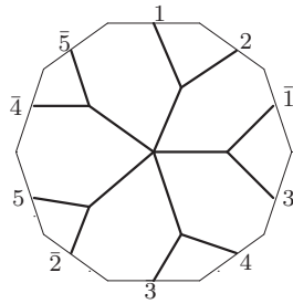
W_6 : o2 - 08 - 40
