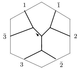
W_4 : o0 - 01 - 01
