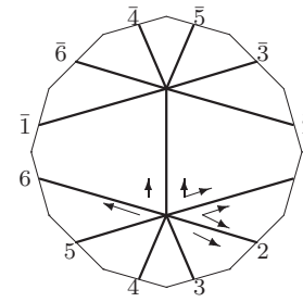
L_7 : o2 - 21 - 07
