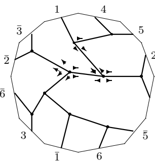
C_{15,11} : o2 - 05 - 15
