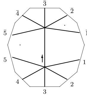
L_6 : o0 - 01 - 01
