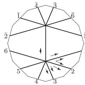
L_7 : o1 - 05 - 07
