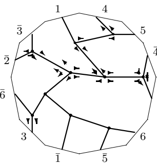
C_{15,11} : o2 - 08 - 30
