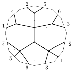
K_{4,3} : o2 - 10 - 48
