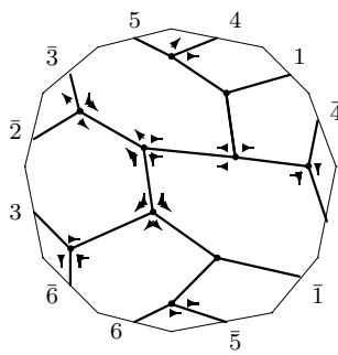
C_{15,11} : o2 - 04 - 30
