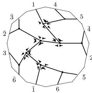
C_{15,11} : o3 - 10 - 30
