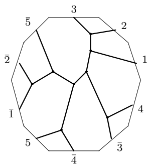
C_{12,1} : o2 - 04 - 48
