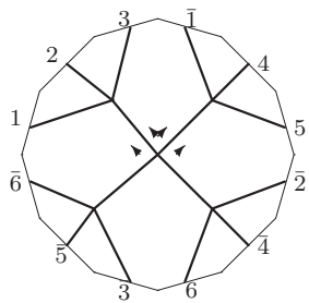
K_5 : o2 - 01 - 04
