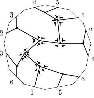
C_{15,11} : o2 - 26 - 30
