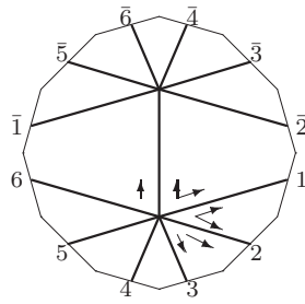
L_7 : o2 - 19 - 07
