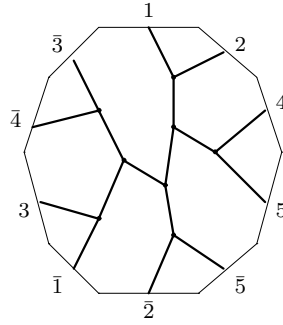
C_{12,2} : o2 - 05 - 48
