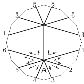
L_7 : o2 - 10 - 14
