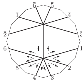
L_7 : o1 - 06 - 14
