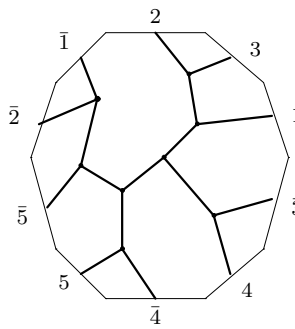
C_{12,1} : o1 - 07 - 48
