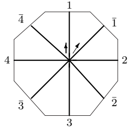
B_4 : o0 - 01 - 02
