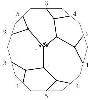
C_{12,3} : o2 - 13 - 03
