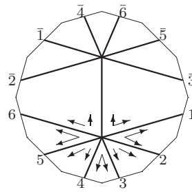
L_7 : o2 - 23 - 14
