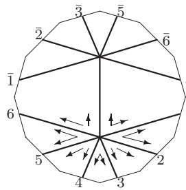
L_7 : o3 - 02 - 14
