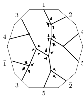
C_{12,2} : o2 - 03 - 24
