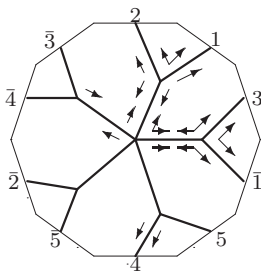
W_6 : o2 - 34 - 20
