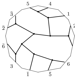
C_{15,11} : o3 - 01 - 60
