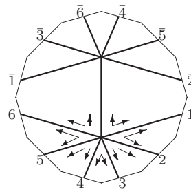
L_7 : o3 - 08 - 14
