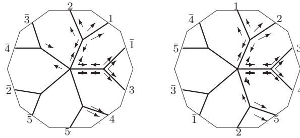
W_6 : o1 - 13 - 20
