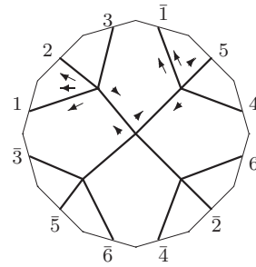
K_5 : o3 - 09 - 10
