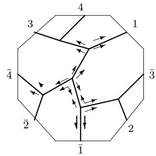
C_{9,1} : o2 - 02 - 18
