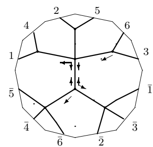
K_{4,3} : o3 - 03 - 08
