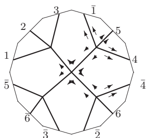
K_5 : o1 - 02 - 20
