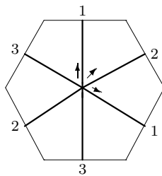
B_3 : q3 - 07 - 03
