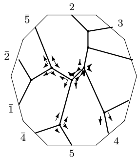
C_{12,1} : o2 - 10 - 48
