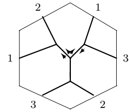
W_4 : q3 - 03 - 04
