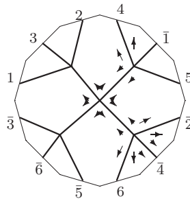
K_5 : o3 - 13 - 20
