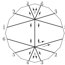
L_7 : o3 - 03 - 14
