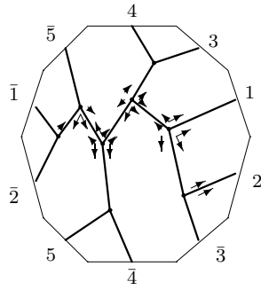
C_{12,1} : o1 - 14 - 24
