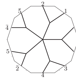
W_6 : o1 - 06 - 40
