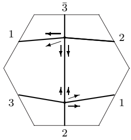
L_4 : q3 - 01 - 08
