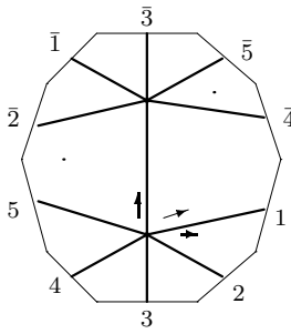
L_6 : o1 - 03 - 03
