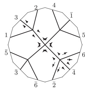
K_5 : o2 - 27 - 20
