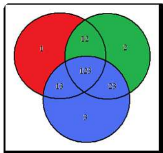
Figure II.1. Cadre de discernement généralisé pour n = 3
